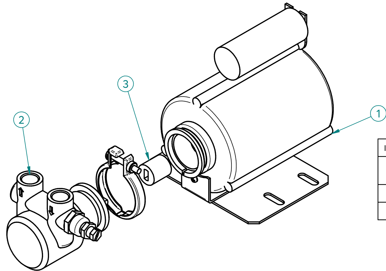
32 - PM_MOTOR BOMBA VELA CONJ. 32 - PM_MOTOR PUMP VELA ASSEMB.
